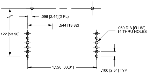
P.C. FOOT PRINT
